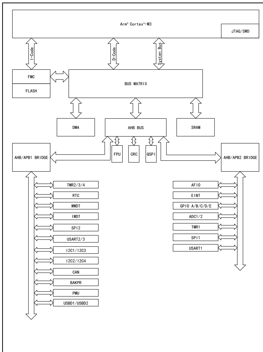
图 1 APM32F103x4x6x8xB 系列产品系统架构
