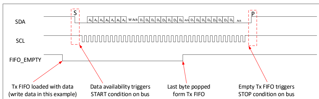
图 86 “TXFIFO 在作为主发送器”I2C 时序图
