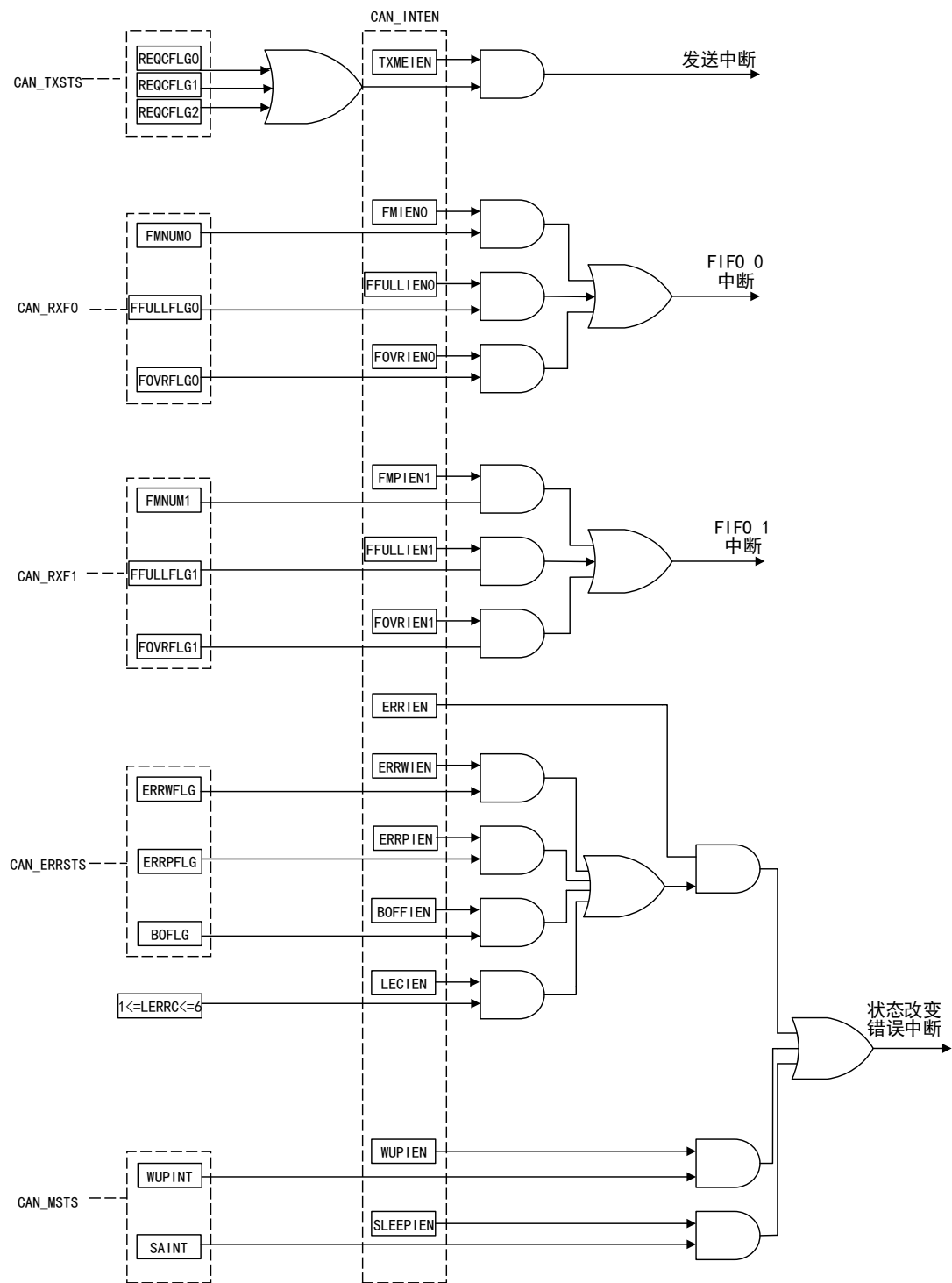
图 109 事件标志和中断产生
