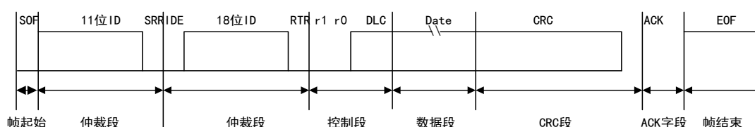
图 102 扩展数据帧
