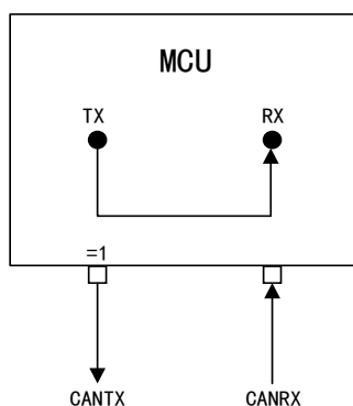
图 105 CAN 工作在静默环回模式
